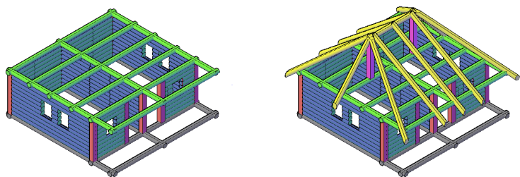
Fig. 2 – Reconstituirea casei lui Ioan Neculae Matei din Costești-Vâlsan, 1860. Varianta II, cu structură de comandată.
