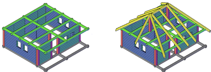
Fig. 1 – Reconstituirea casei lui Ioan Neculae Matei din Costești-Vâlsan, 1860. Varianta I, cu structură nedecomandată.
