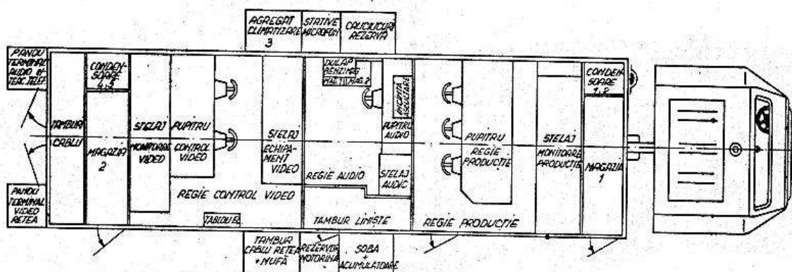
SCHEMĂ AMPLASARE
